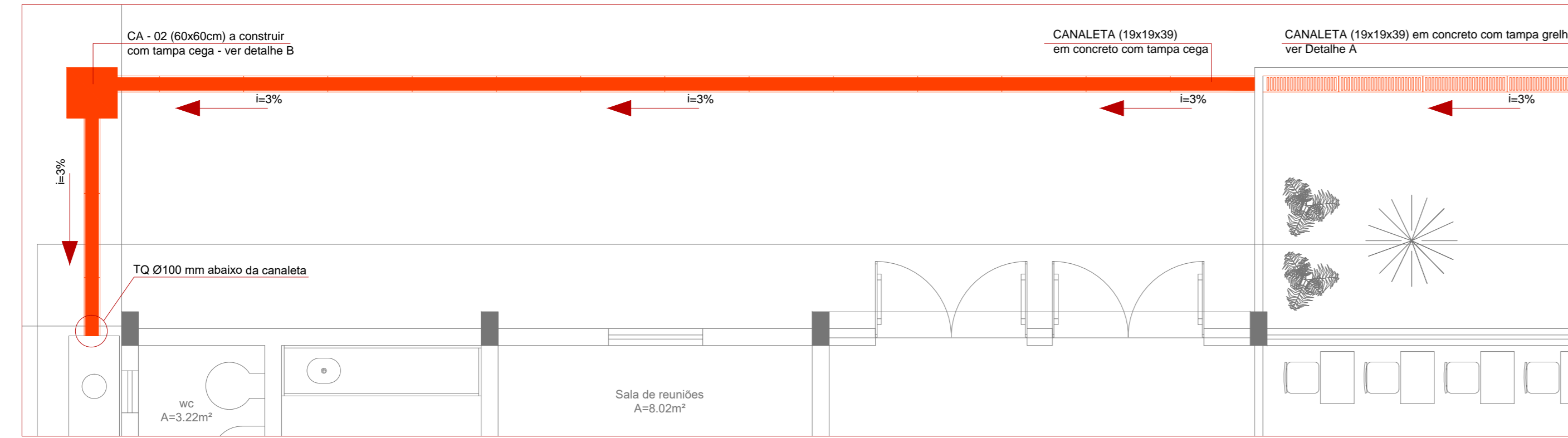
Planta Baixa Hidrossanitário Esgoto Pluvial - Detalhe n° 01A ESCALA: 1/50
