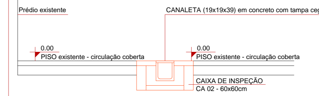
Detalhes B ESCALA: 1/75
