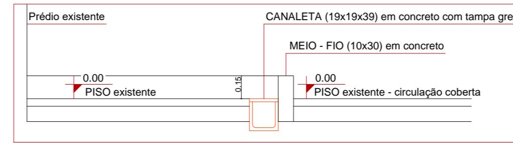
Detalhes A ESCALA: 1/25
