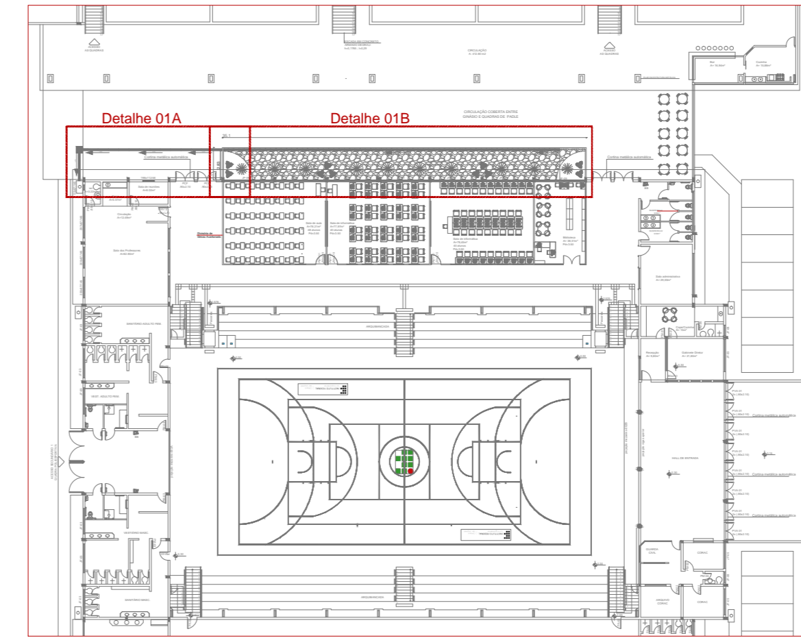
Planta Baixa Geral - Localização Detalhes ESCALA: sem escala
